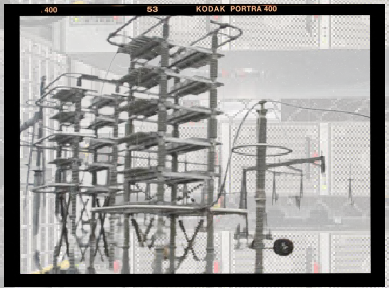
Capacitor Set
